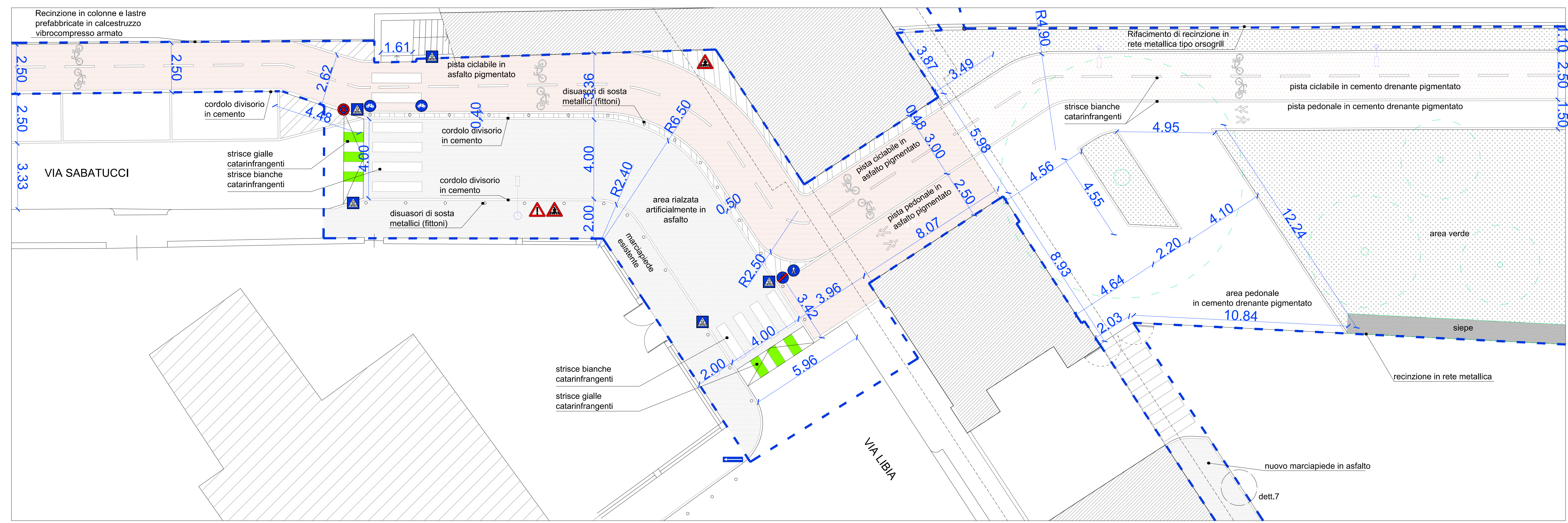
pianta area sotto il ponte di via Libia scala 1:100
